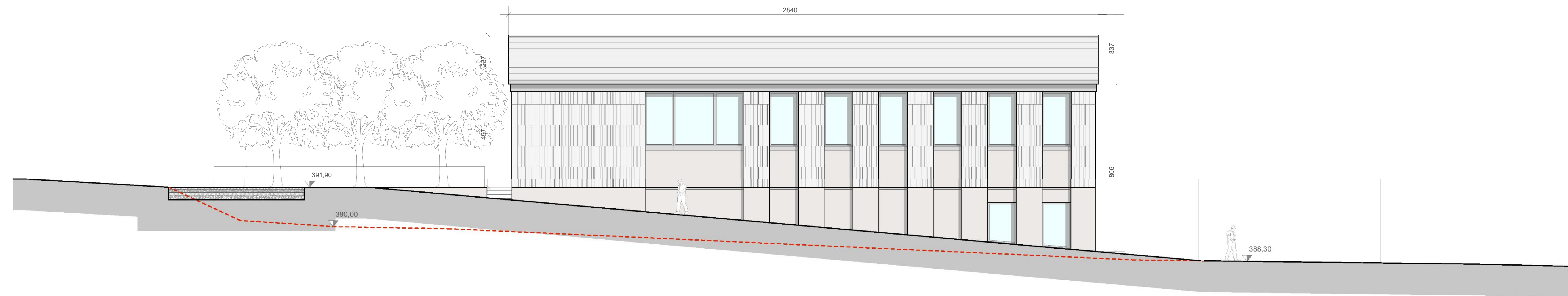
SEZIONE BB'
