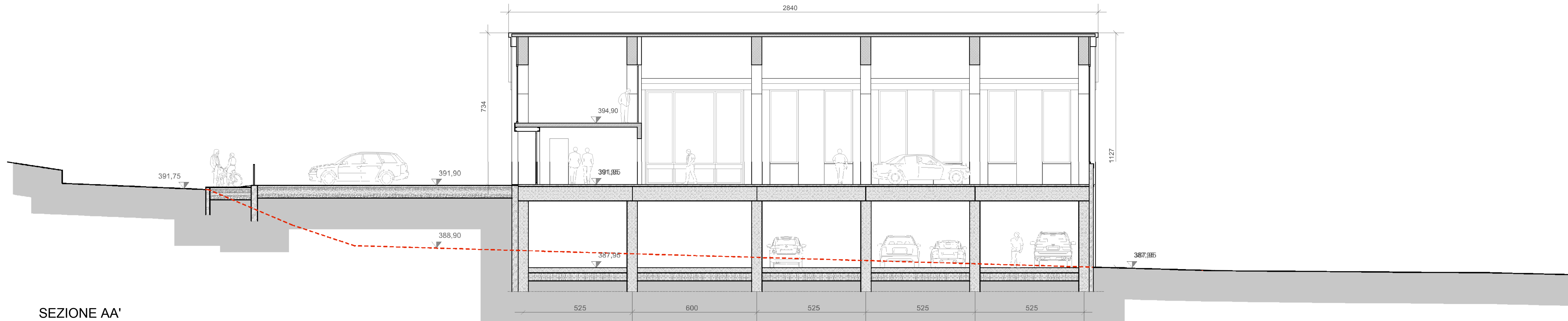
SEZIONE AA'
